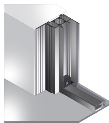
D: Montage im lichten Maß mit Montageprofil schmal
